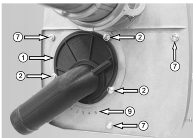
Fig. 4: Pezzo di raccordo RLU montato
