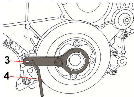
Herramienta de alineación del cigüeñal (3/4)
