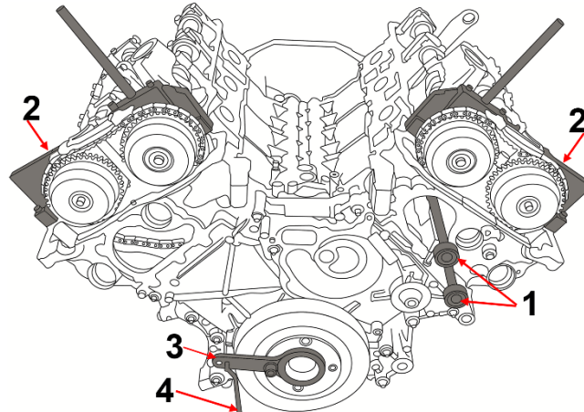
Herramienta de alineación del cigüeñal (3/4)
