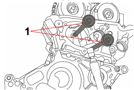
Herramienta tensora de cadena de distribución (1)
