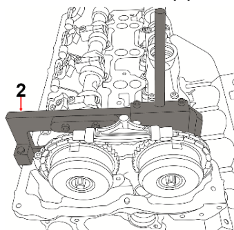
Herramientas de ajuste del árbol de levas (2)
