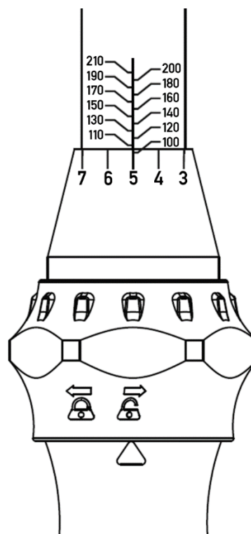
Ejemplo 105 Nm
