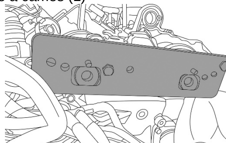
Kit d'outils de verrouillage d'arbre à cames (1)
