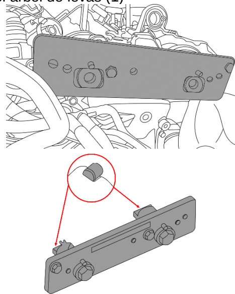
Juego de herramientas de bloqueo del árbol de levas (1)
