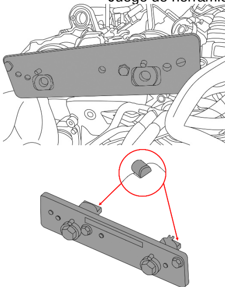
Juego de herramientas de bloqueo del árbol de levas (1)
